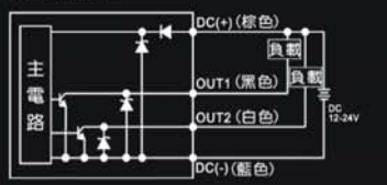
EP42□-02-□-□ NPN 輸出
