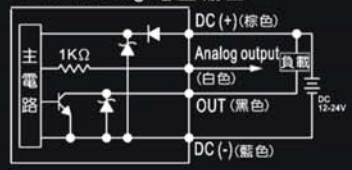
EP42□-010-□-□ NPN+Analog 電壓輸出
