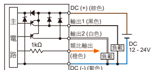
EP8 □ - 030 - M5 2 PNP + 類比電壓輸出 (1 ~ 5 V)
