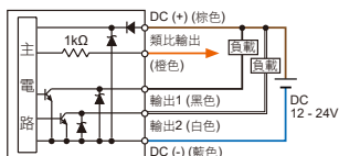
EP8 □ - 010 - M5 2 NPN + 類比電壓輸出 (1 ~ 5 V)
