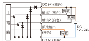
EP8 □ - 011 - M5 2 NPN + 類比電流輸出 (4 ~ 20 mA)
