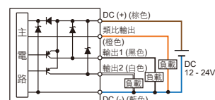
EP8 □ - 031 - M5 2 PNP + 類比電流輸出 (4 ~ 20 mA)
